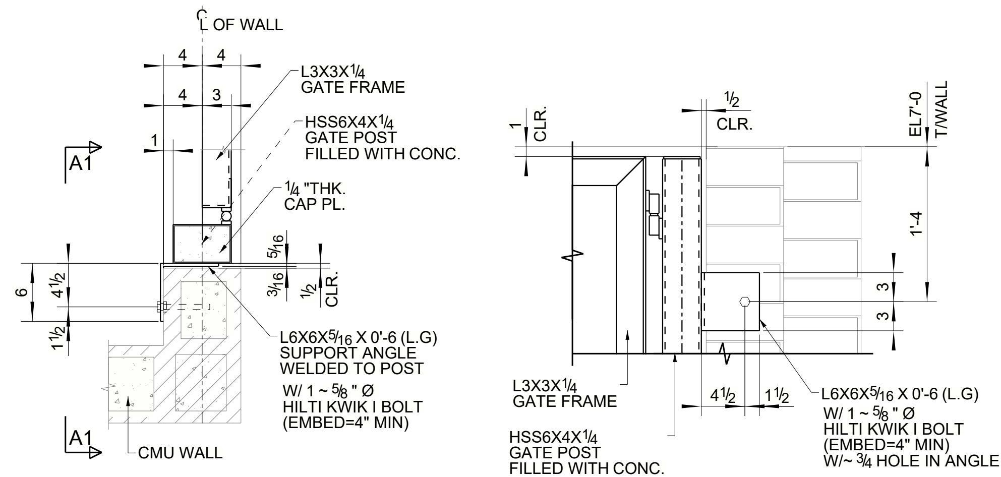
DETAIL A E11
