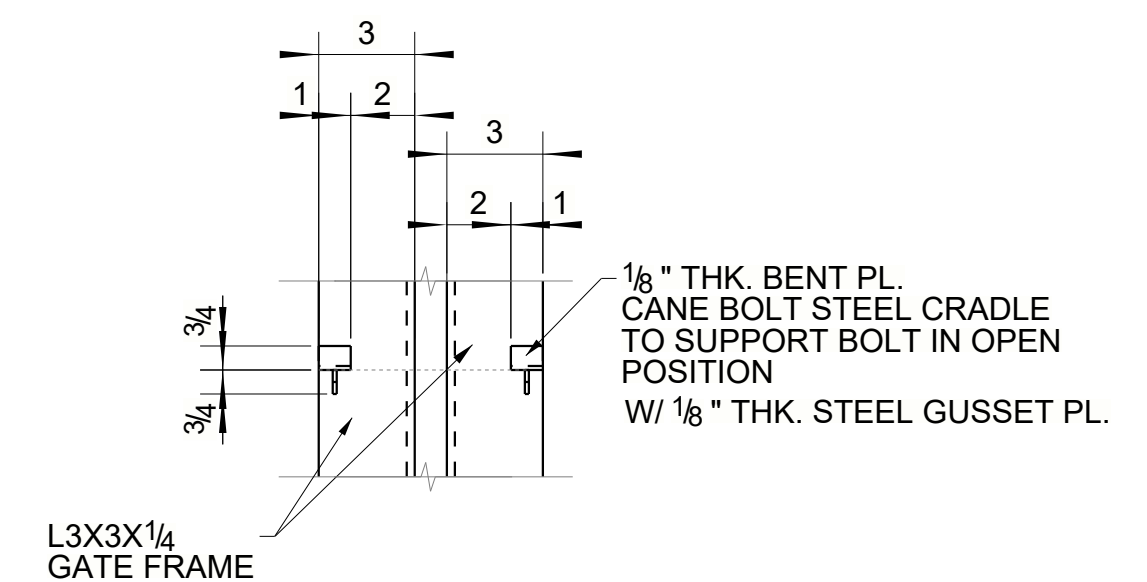
SECTION A1 - A1
