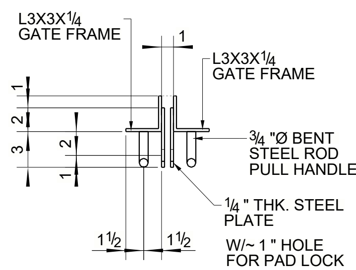
SECTION B3 - B3
