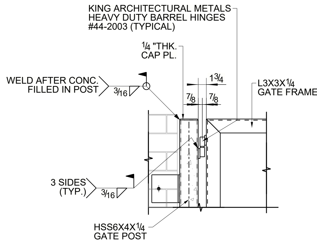
DETAIL C E12
